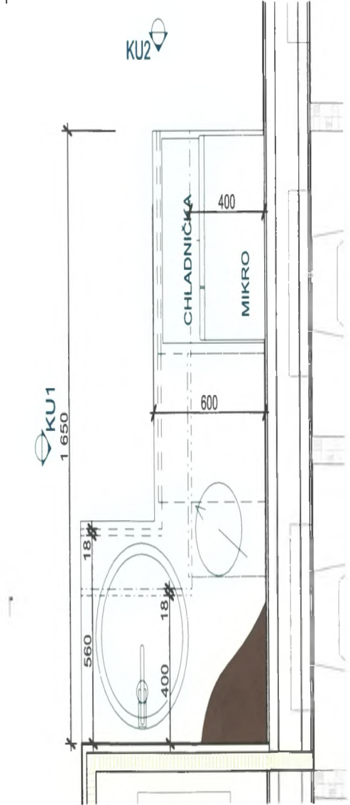
PŮDORYS 1.NP - KUCHYŇSKÁ LINKA 1:20
