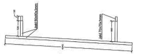
Rám 2
