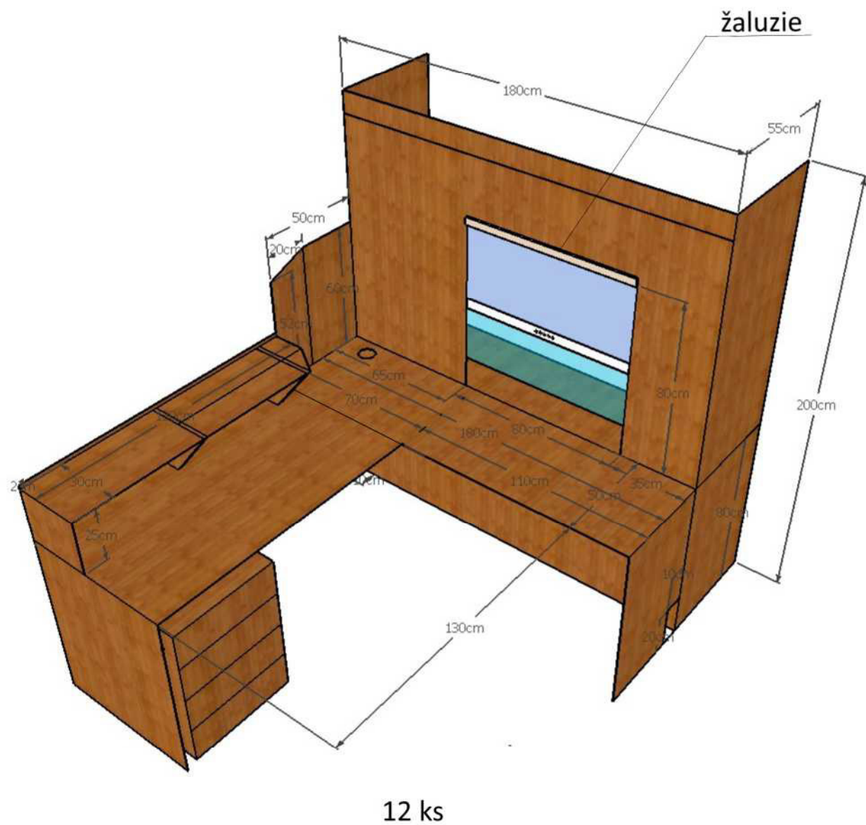
Př. č. 2 - Přepážka 180 cm (standardní)
