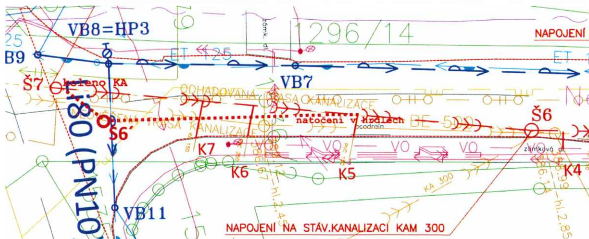
Úsek změny trasy kanalizace
