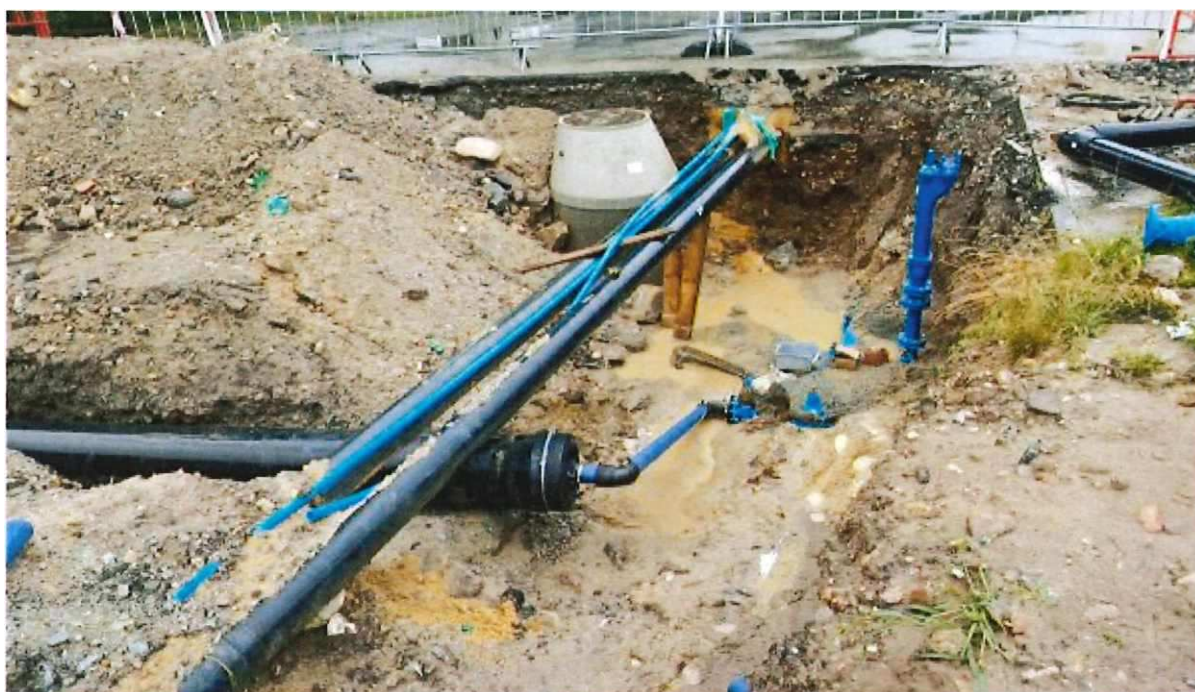
Provádění shybky
