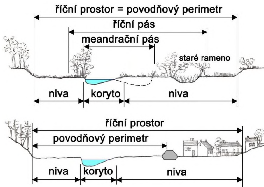
Obr. 69: Členění říčního prostoru meandrujícího vodního toku v ploché nivě. Nahoře přirozené podmínky povodňových rozlivů. Dole jsou rozlivy omezeny ochranným ohražováním zastavěné části nivy. Převzato z Just a kol. (2020).
