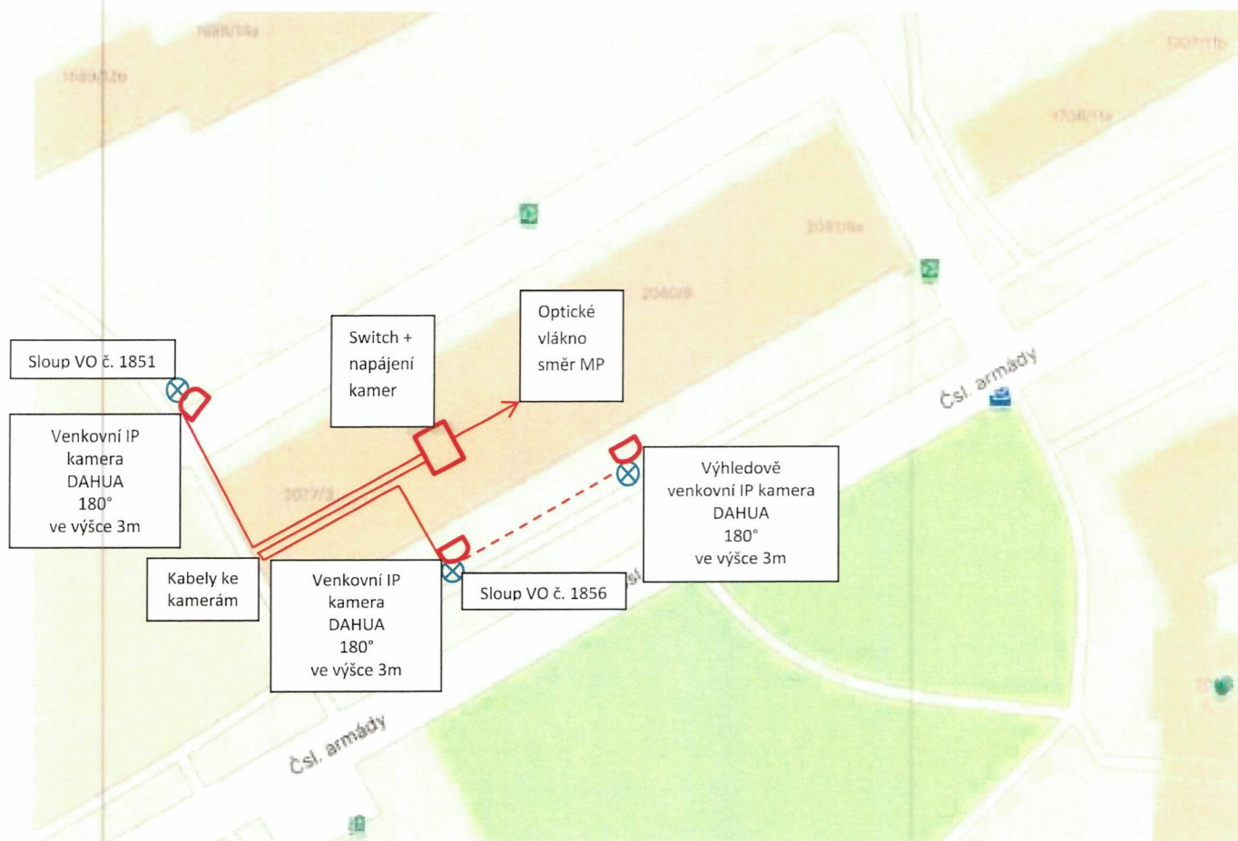
Schéma rozmístění kamer a kabelů na objektu Čsl. Armády 3, Šumperk.
