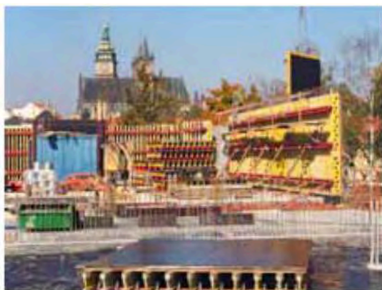
(25) Obr. F.4 – Nosníkové bednění
