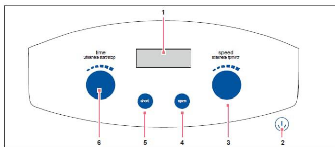
Obr. 5-1: Ovládací prvky obsluhy centrifugy 5702
