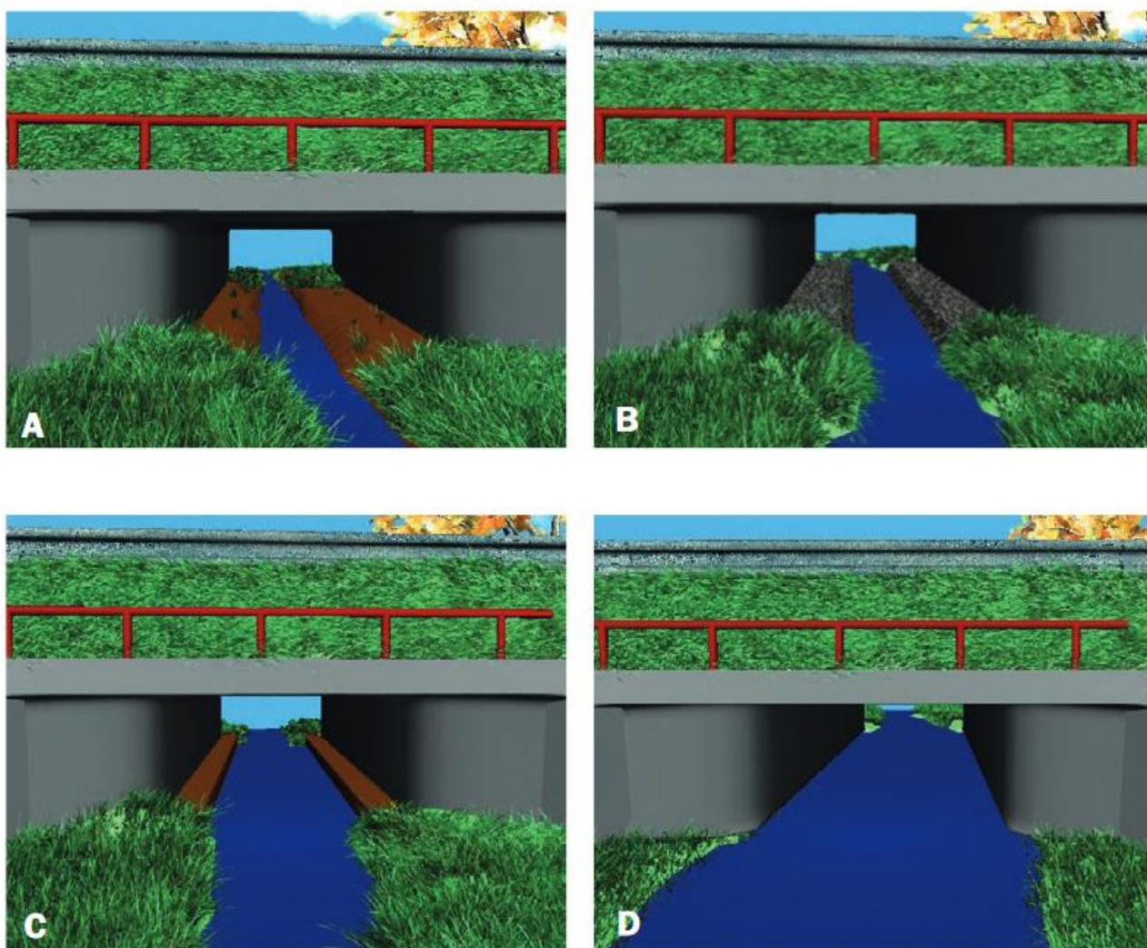
Obr. 51: Různé varianty zajištění suchých břehů pod mostem pro průchod vydry: A - přirozené břehy (optimální situace), B – kamenné postranní bermy (přijatelné řešení), C – zdivé či dřevěné postranní lávky (mezní řešení) a most bez suchých břehů v podmostí (neakceptovatelné řešení) (D). Převzato z metodiky Vydra a doprava (Hlaváč a kol., 2017).
