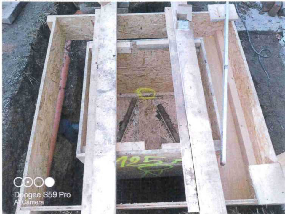
Stav na lokalitě, příprava betonáže jímky (máchadla), zdroj: Zhotovitel
