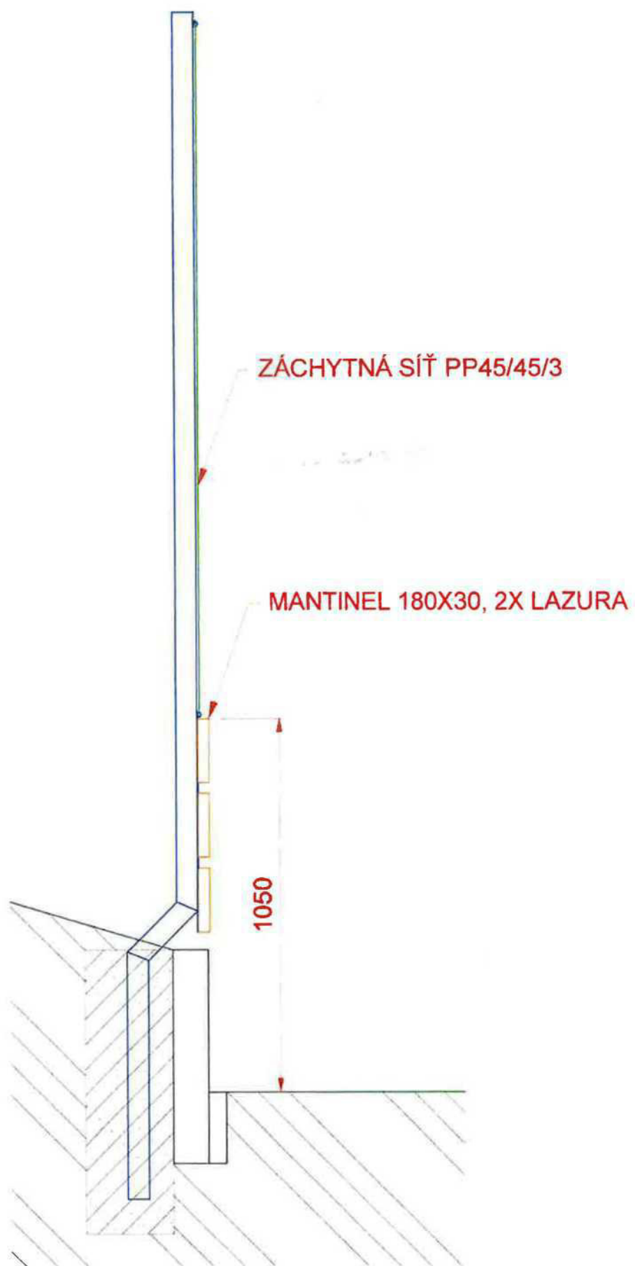
DETAIL - SLOUP LOMENÝ ZA PALISÁDOU
