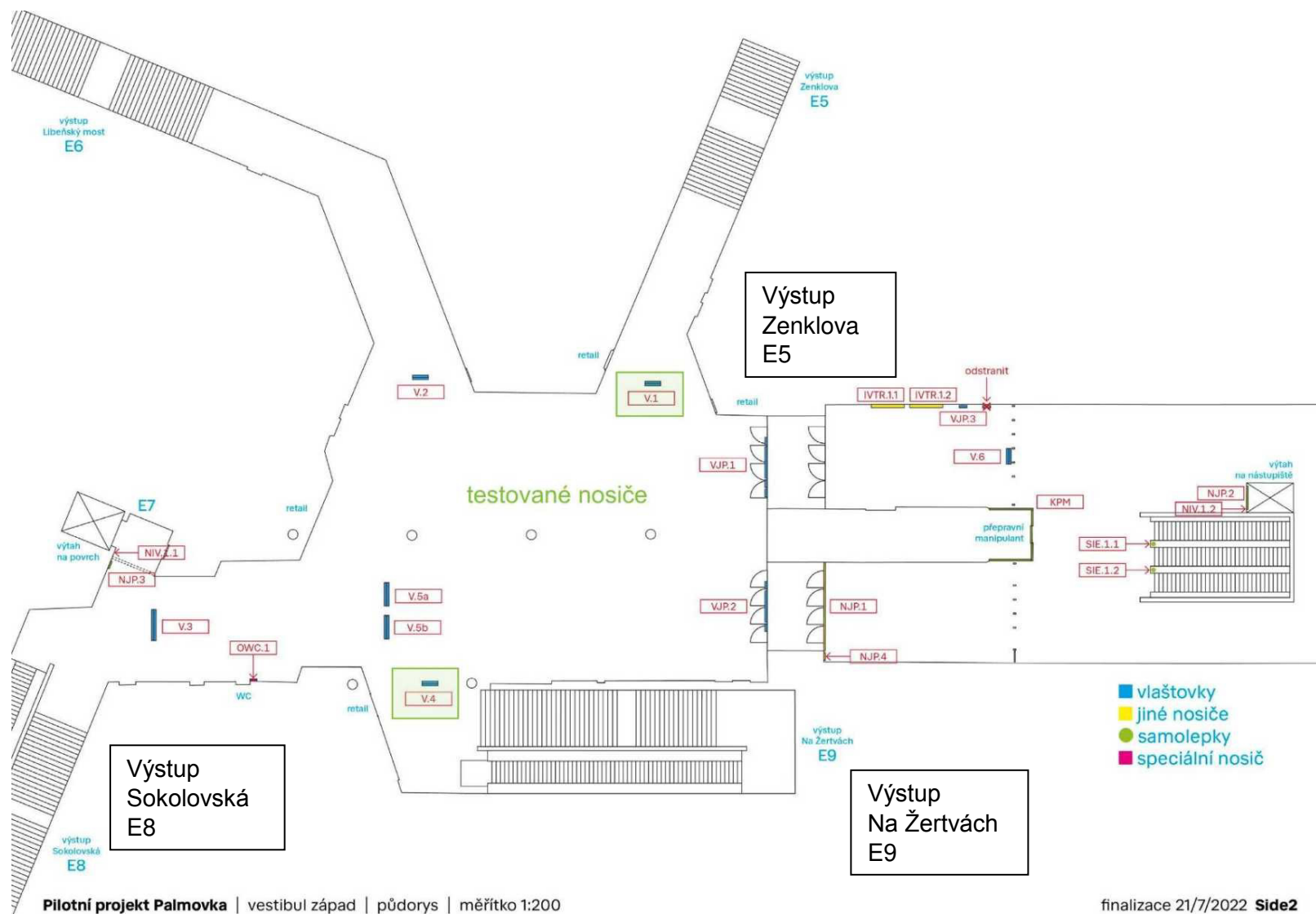
Obrázek 1 Půdorys západního vestibulu stanice Palmovka
