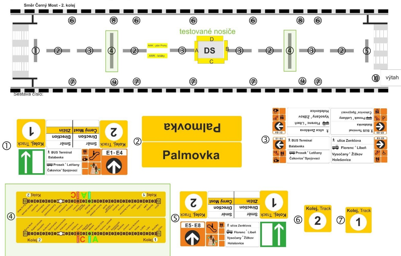
Obrázek 6 Půdorys prostoru nástupišť stanice Palmovka
