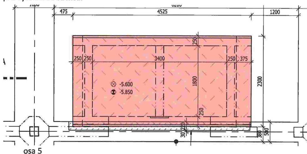
Půdorys výtahové šachty
