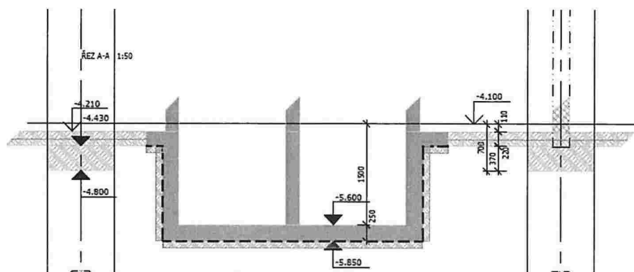
Řez výtahovou šachtou – dojezd
