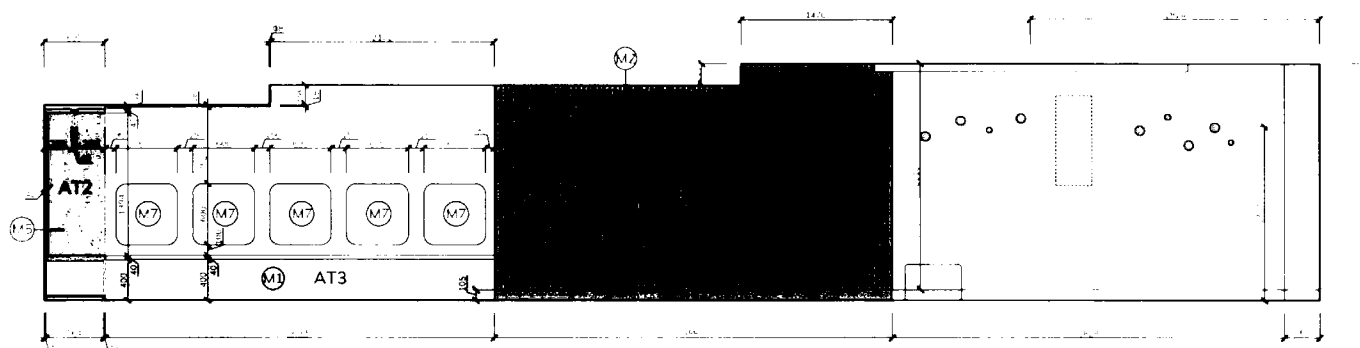
POHLED P2
