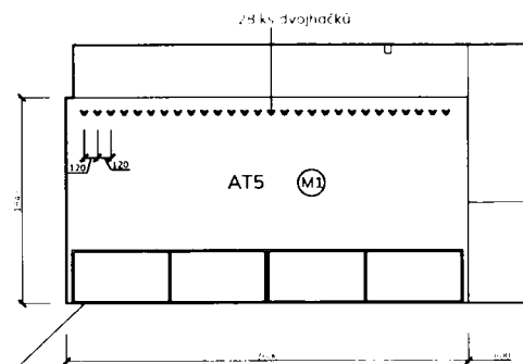
POHLED P6
