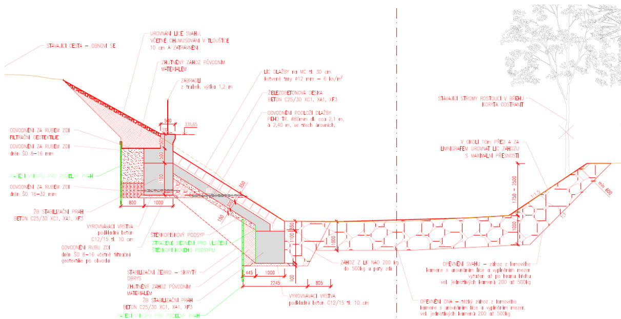
Obr. 1 – Původní vzorový příčný řez korytem Křetínky – varianta ŽB deska obložená kamenem + kamenný zához
