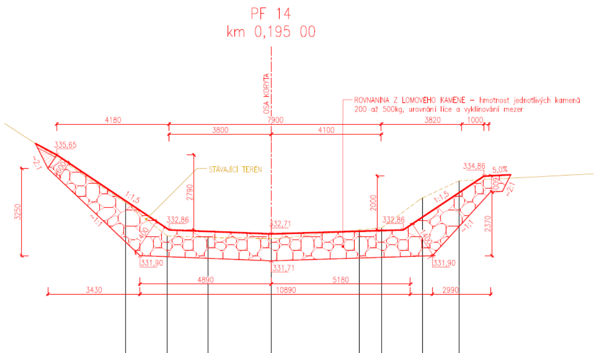
Obr. 2 – příčný řez korytem Křetínky – varianta rovnanina z lomového kamene ve všech částech koryta
