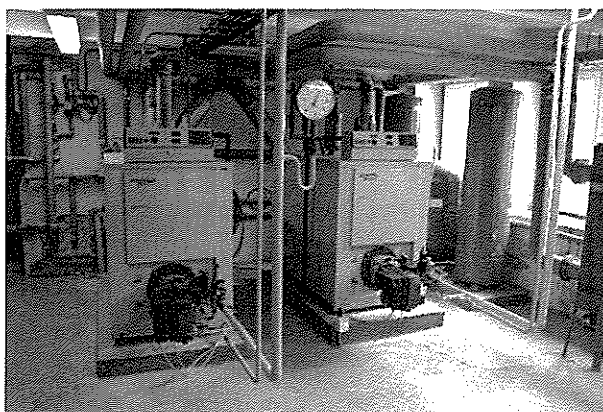
Obrázek 10 - Zdroje tepla
