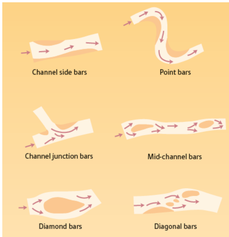
Obr. 63: Typy lavic: střídavé (i v upravených korytech, nejméně stabilní), zákrutové (jesepní), výústní (přítok přináší sediment), střední (málo stabilní, zpravidla za překážkou), diamantové (stabilnější, může se uchytit i vegetace), příčné (narušení diamantových); obrázek převzat z Holden (2017)
