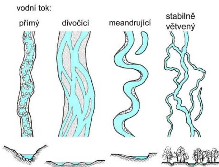
Obr. 5: Geomorfologické typy vodních toků podle půdorysných tvarů koryta (Just, 2005)
