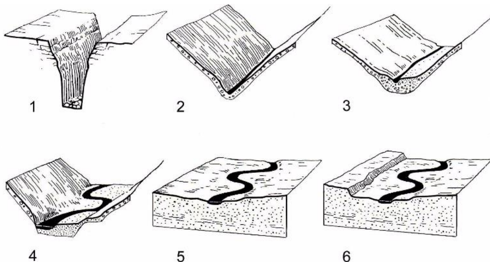
Obr. 12: Typy údolí: 1 – soutěska tvaru hlubokého U (vysoká E toku, odnos horninového materiálu); 2 – zařiznuté údolí tvaru V (koryto zásobováno materiálem ze svahů, který omezuje pohyb do stran); 3 – kotlina s přímým nebo divočícím korytem (dostatek materiálu, E nestačí na jeho odnos ani pohyb do stran); 4 – údolí s meandry ( neckovitě ); 5 – plochá niva ( úvalovitě ); 6 – plochá niva se starší terasou (Just, 2005, upraveno podle Kerna, 1994)
