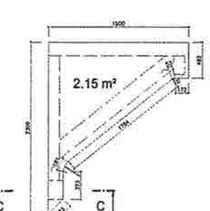
ŘEZ C-C
