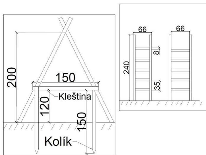
Vyzpěrování - přelez
