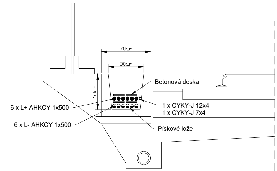
VZOROVÝ ŘEZ ULOŽENÍ KABELŮ PODEl TRAMVAJOVÉ TRATI - 6xL+/L-
