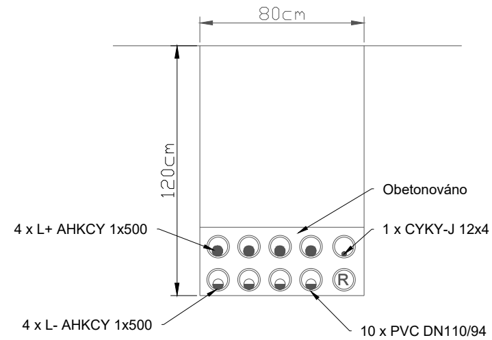
VZOROVÝ ŘEZ ULOŽENÍ KABELŮ POD TRAMVAJOVOU TRATÍ - 4xL+/L-
