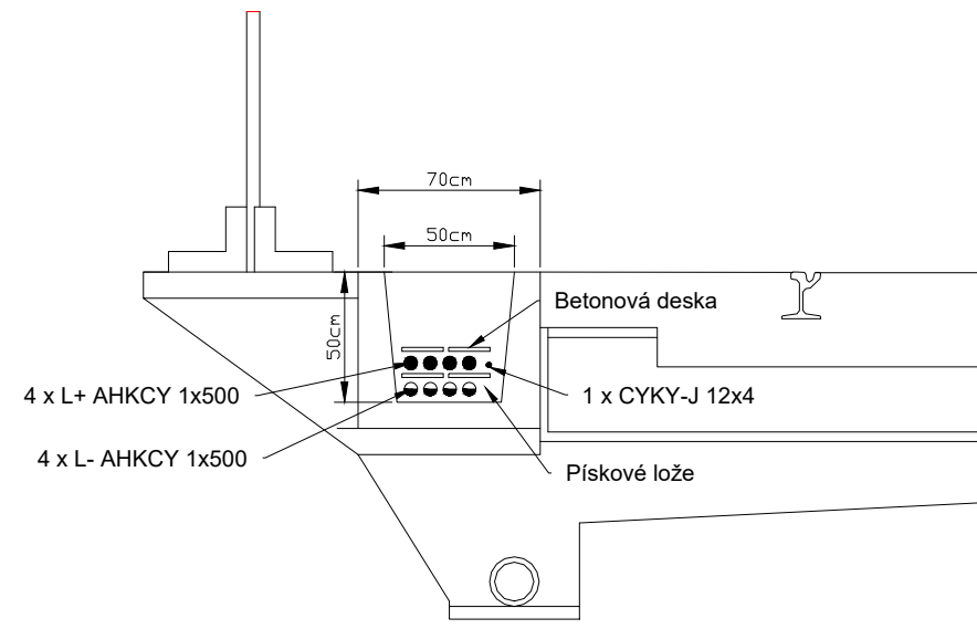
VZOROVÝ ŘEZ ULOŽENÍ KABELŮ PODEl TRAMVAJOVÉ TRATI - 4xL+/L-
