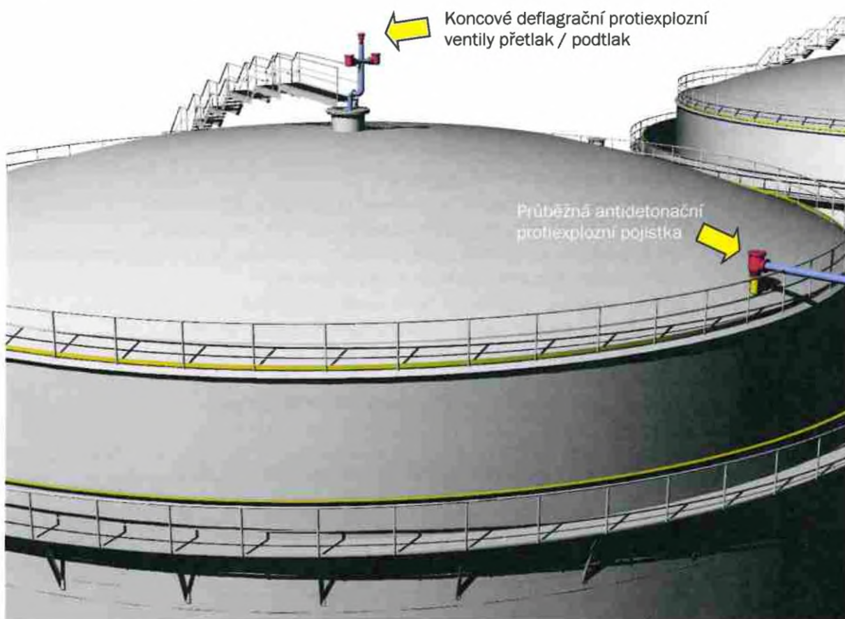
Obr. 1 – Obvyklá technologická instrumentace nádrže BA
