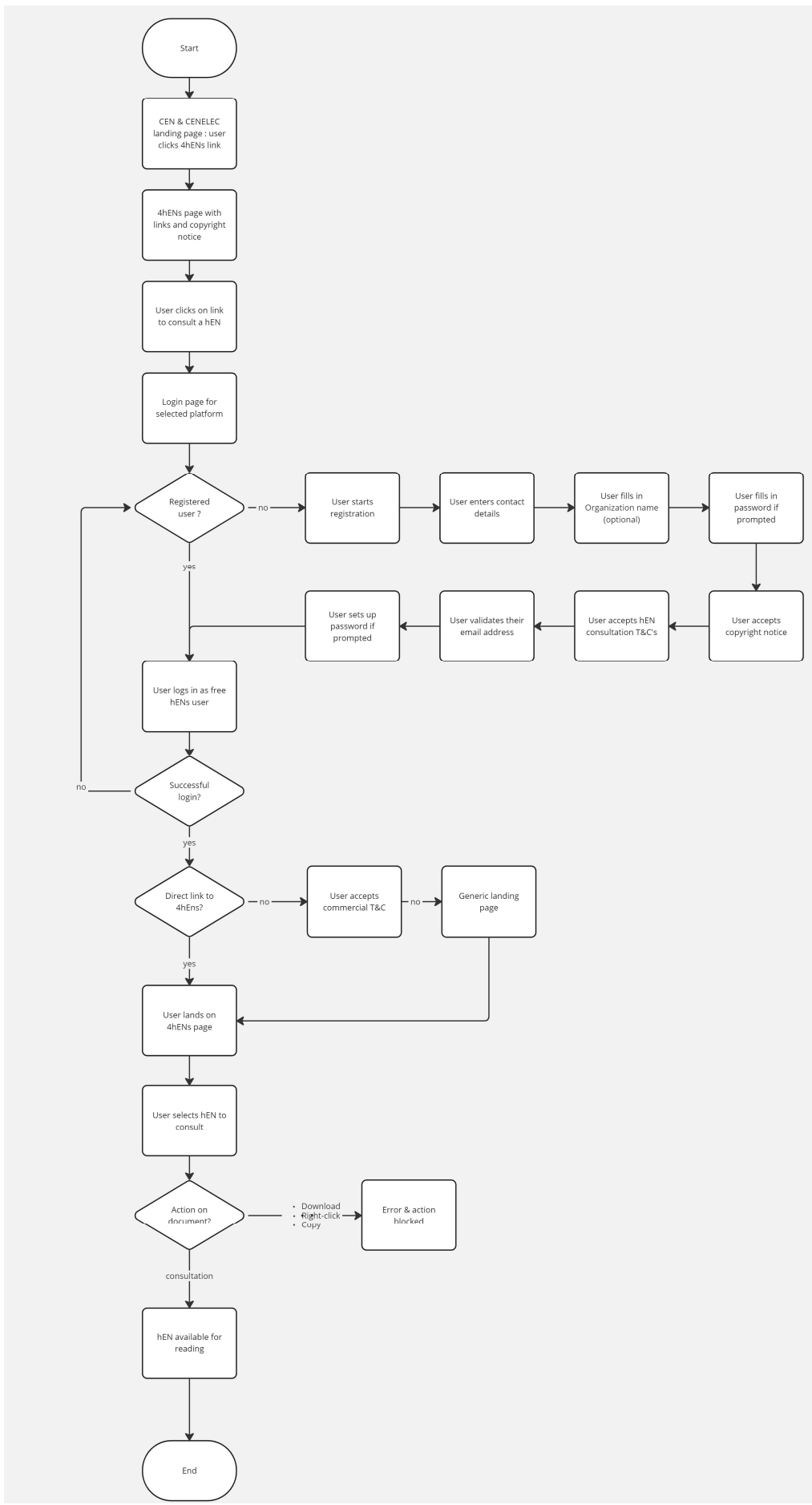
Obrázek 4 - Procesní mapaa
