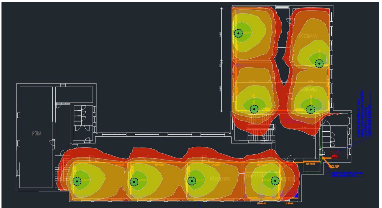
3.NP Síla signálu 5GHz budova ZŠ II. stupeň
