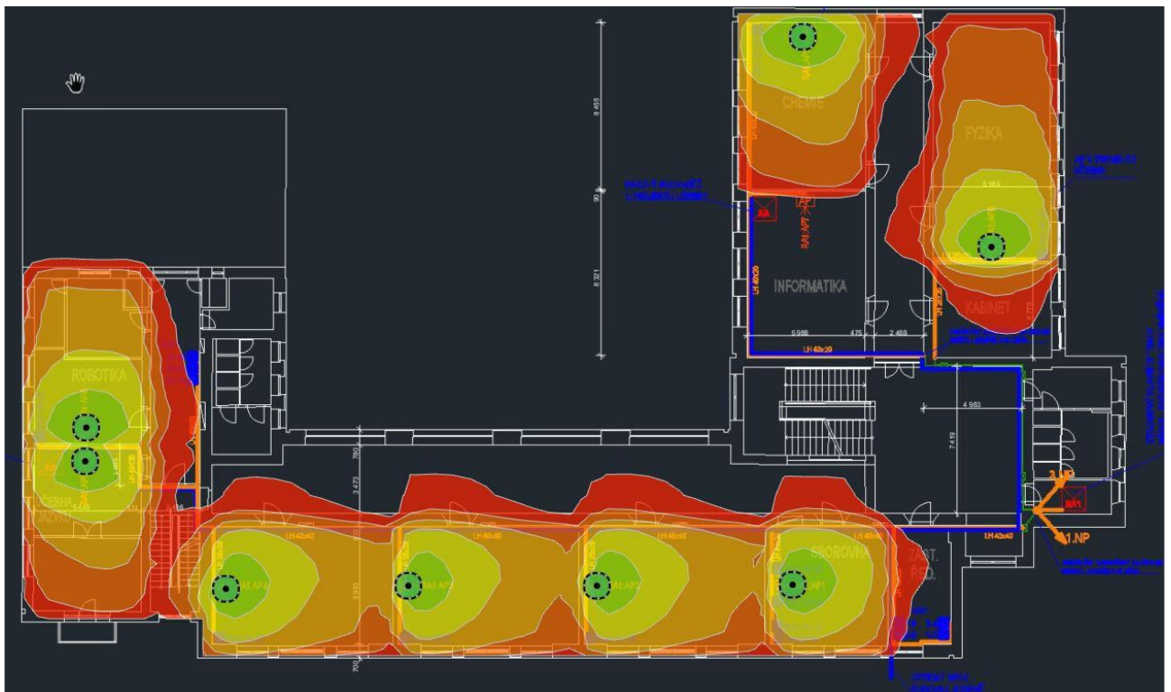
3.NP Síla signálu 2,4GHz budova ZŠ II. stupeň
