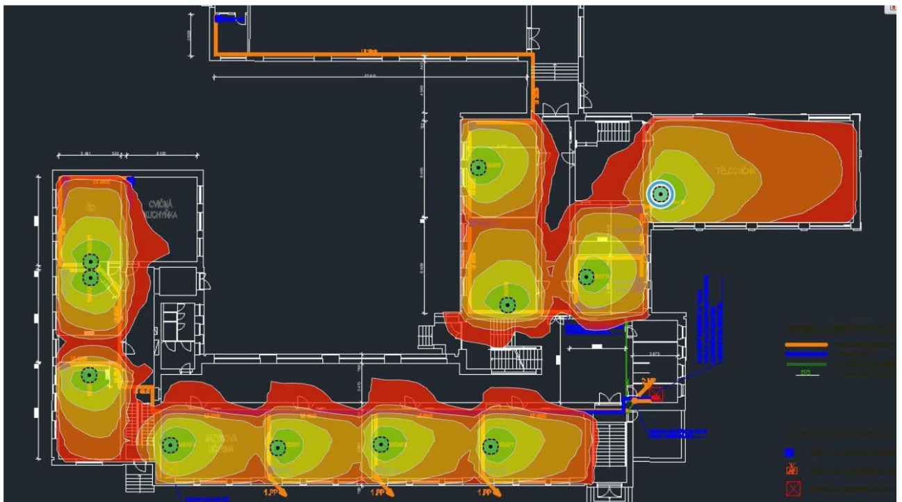
2.NP Síla signálu 2,4GHz budova ZŠ II. stupeň
