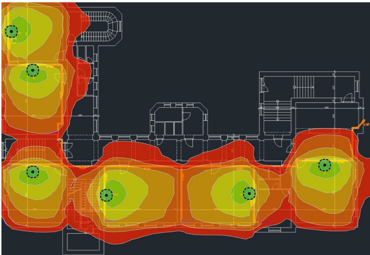
2.NP Síla signálu 2,4GHz budova ZŠ – I. stupeň
