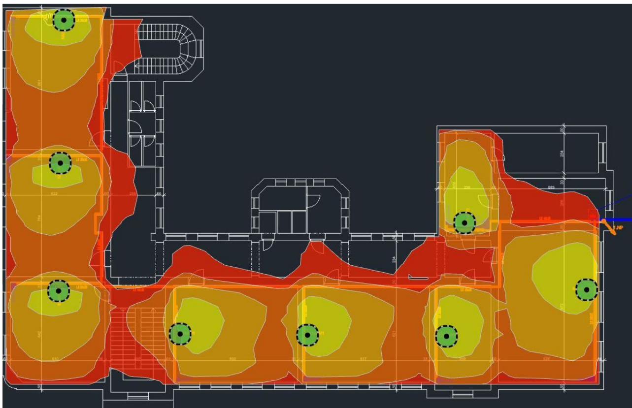
2.NP Síla signálu 5GHz budova ZŠ – I. stupeň
