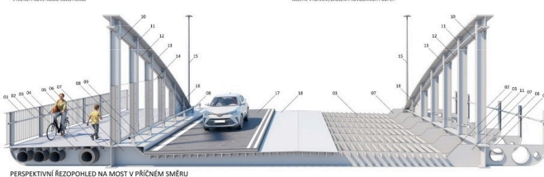
PERSPEKTIVNÍ ŘEZPOHLED NA MOST V PŘÍČNÉM SMĚRU
