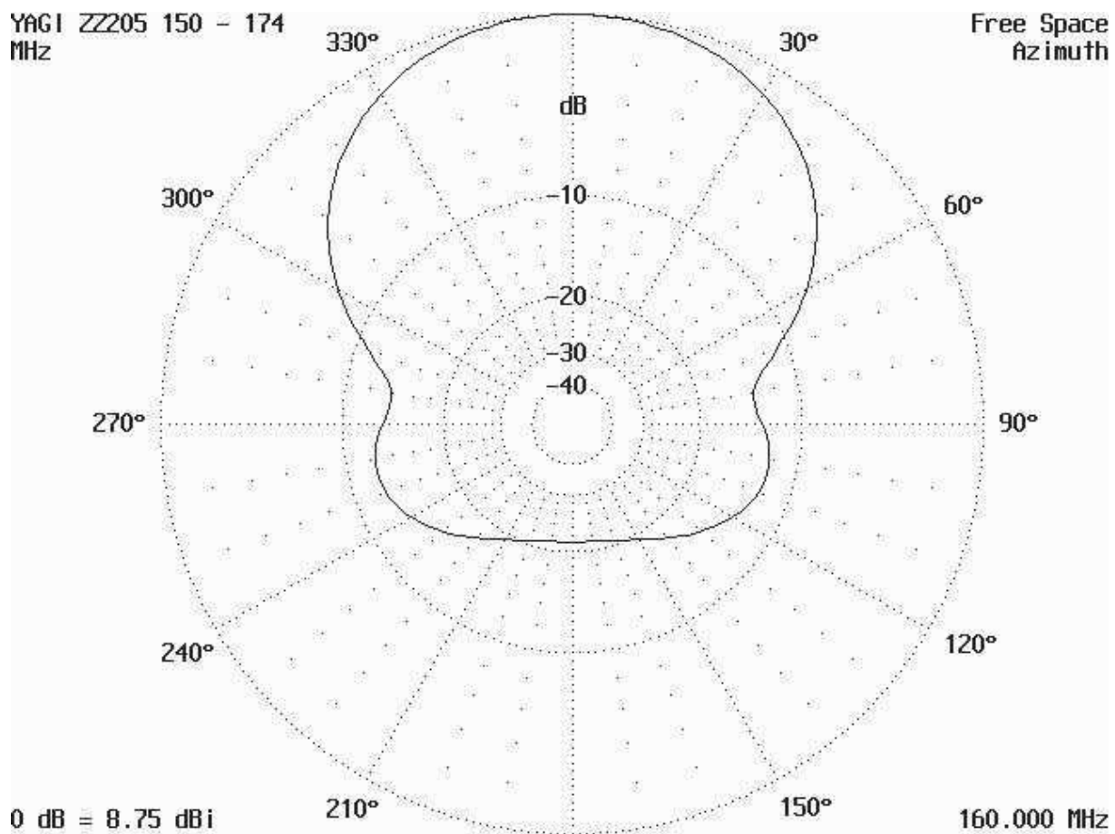
Vyztařovací diagram antény ZZ205 v rovině E
