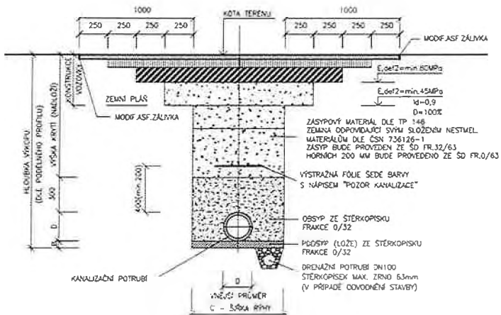
Konstrukce vozovky dle TP 170 D1-N-6-IV-PIII
