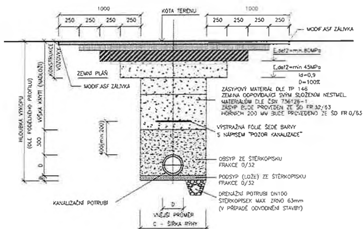
Konstrukce vozovky dle TP 170 D1-N-6-V-PIII
