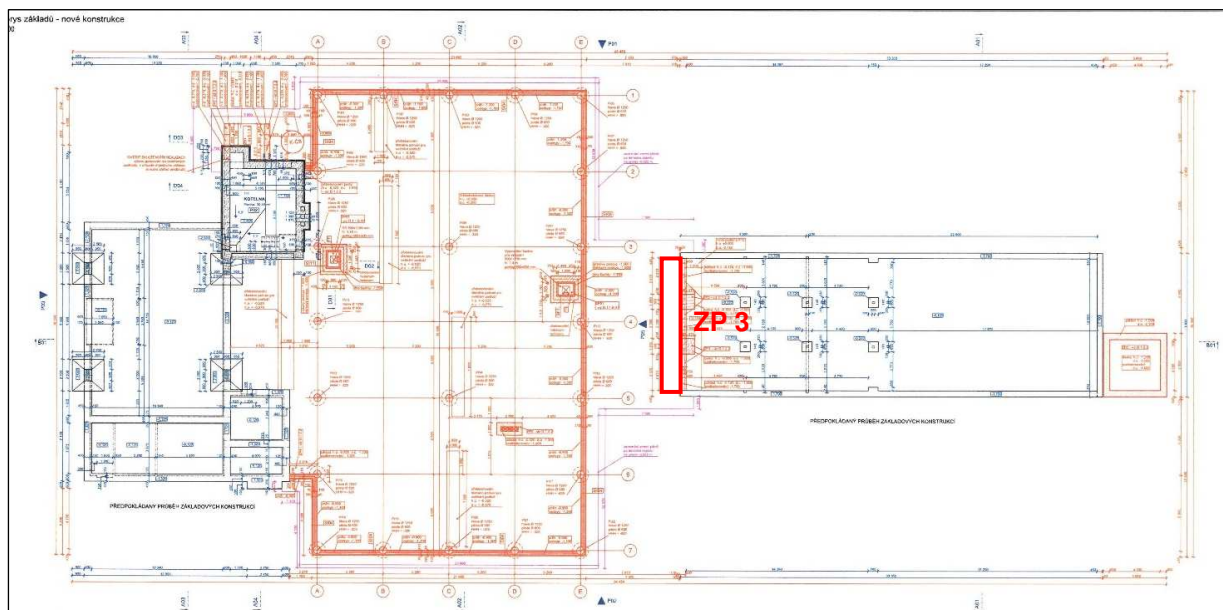
Obr. 1: Situace základové spáry pod základovým pasem nového štítu ZP 3.
