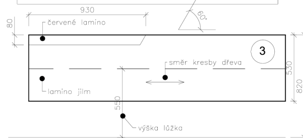
půdorys
