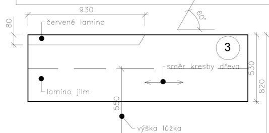
půdorys
