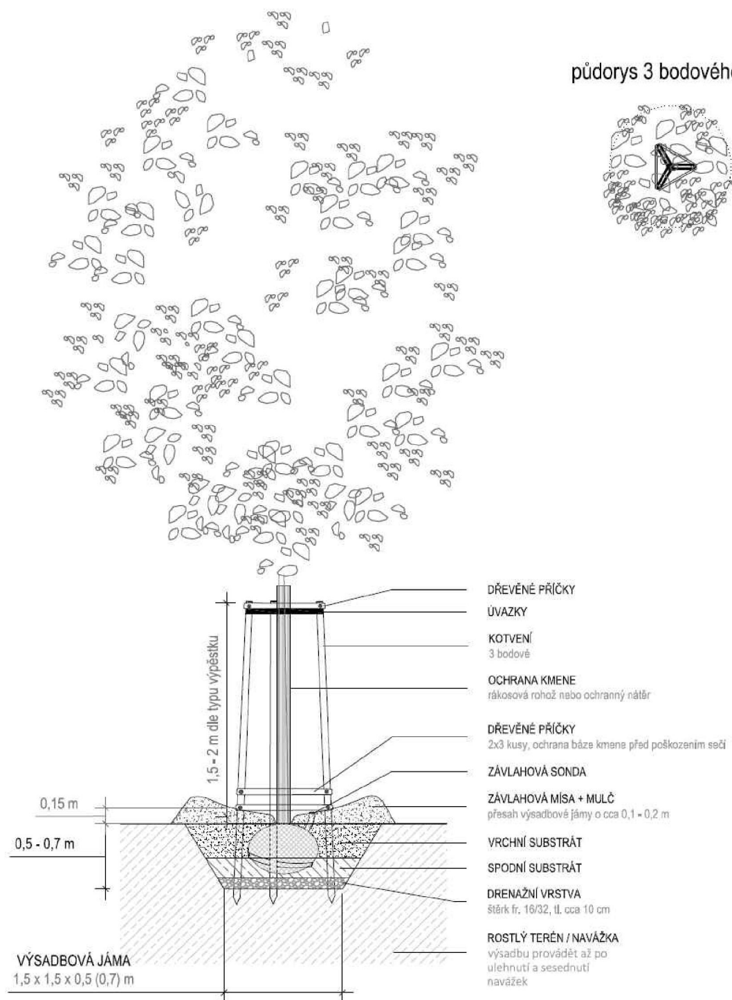
Výsadba stromu – modelové schéma technologie A1
