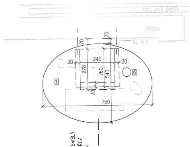
PŮDORYS
