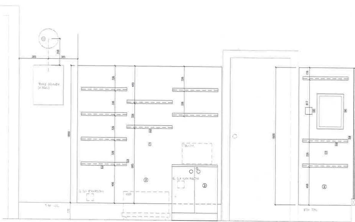
POHLED ČELNÍ
