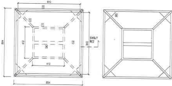
PŮDORYSNÝ ŘEZ
