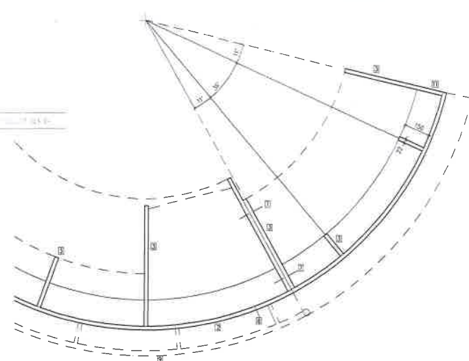
P Ů D O R Y S N Ý Ř E Z 2
