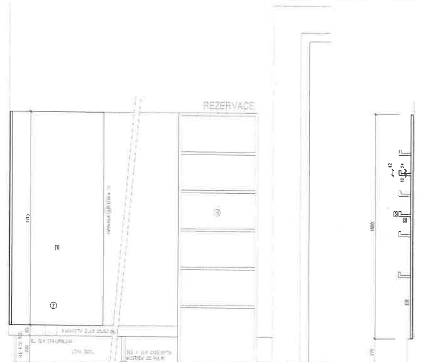
POHLED NA BOČNÍ STĚNU
