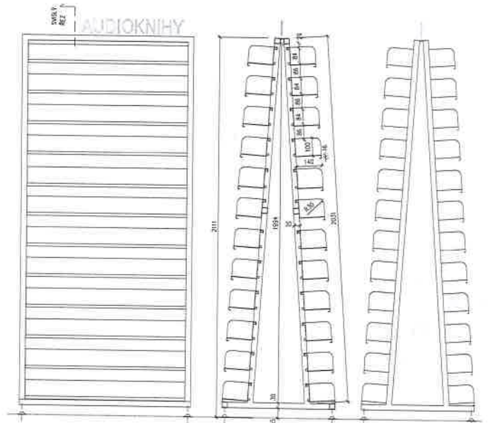
POHLED ČELNÍ
