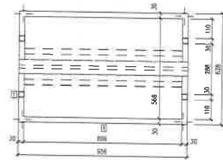
PŮDORYSNÝ ŘEZ – KONSTRUKCE PŘED OSAZENÍM TRNŮ A ZAVĚŠENÍ NOSIČŮ KNIH
