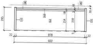
POHLED ČELNÍ
