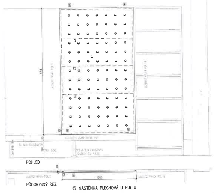
POHLED PŮDORYSNÝ REZ 23 NÁSTĚNKA PLECHOVÁ U PULTU
