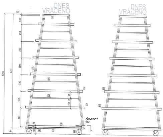
SVISLÝ ŘEZ
