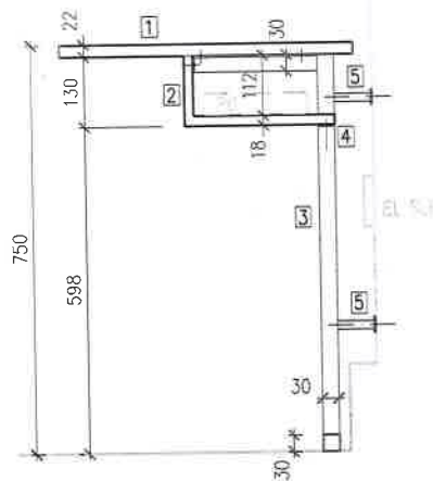
ŘEZ SVISLÝ
