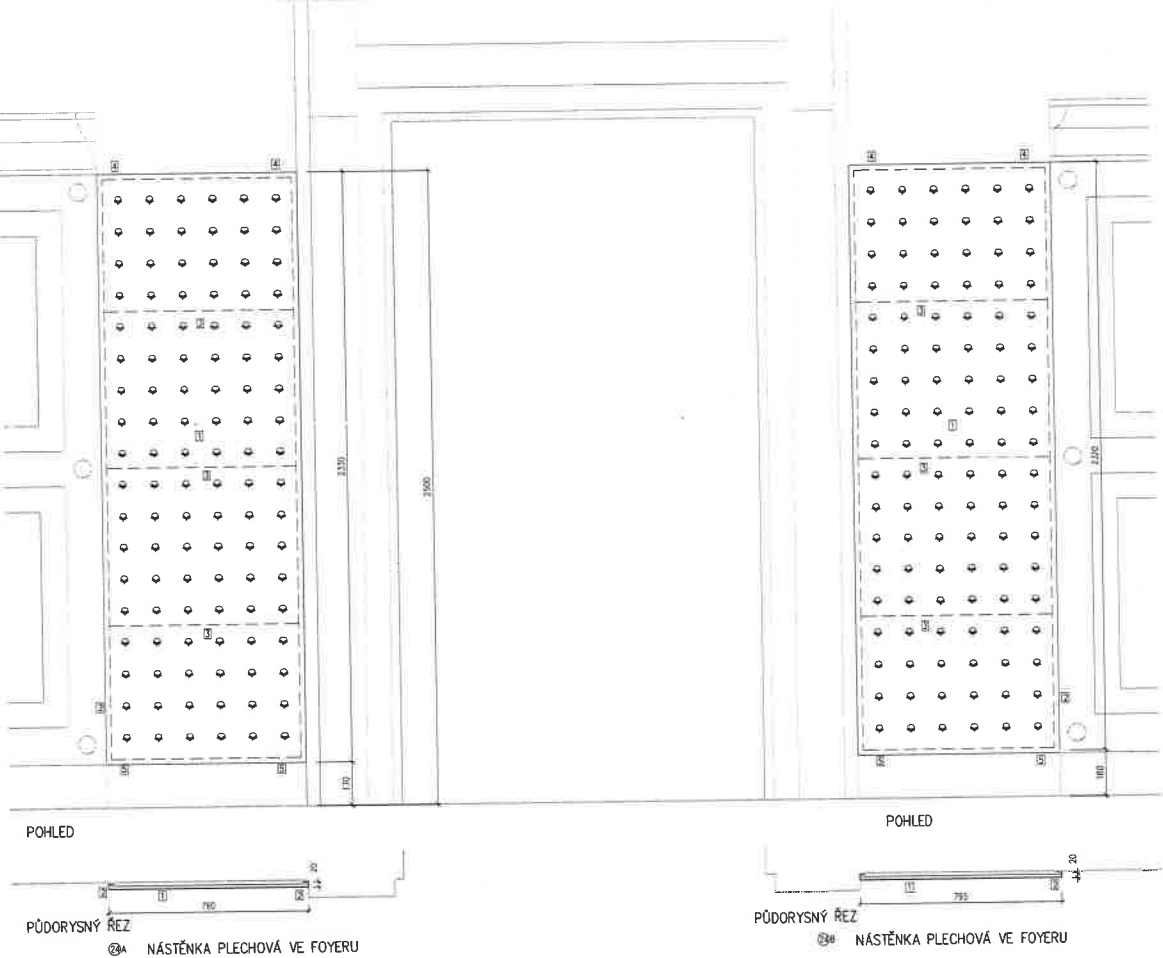
POHLED PŮDORYSNÝ REZ 23a NÁSTĚNKA PLECHOVÁ VE FOYERU POHLED PŮDORYSNÝ REZ 23b NÁSTĚNKA PLECHOVÁ VE FOYERU
