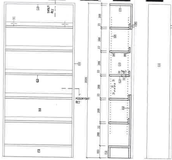
POHLED ČELNÍ
