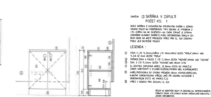
POHLED ČELNÍ
