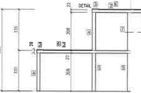
ŘEZ SVISLÝ
