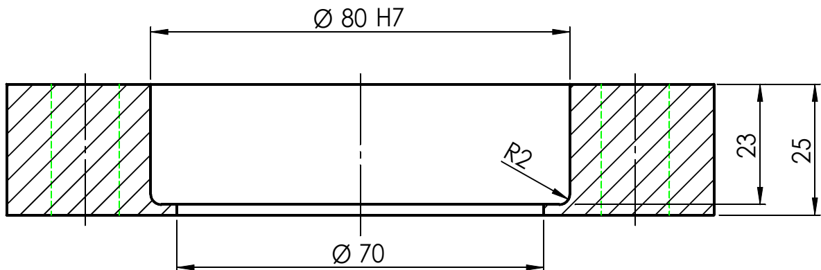
ŘEZ A-A
