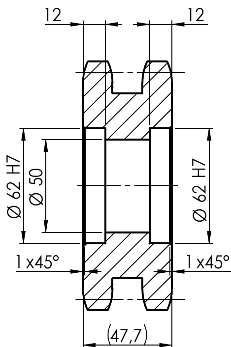
ŘEZ A-A
