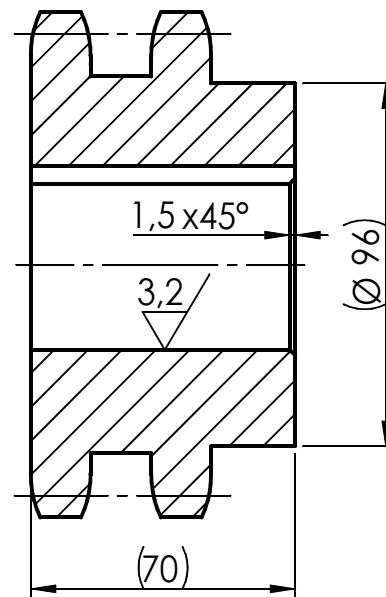
ŘEZ A-A
