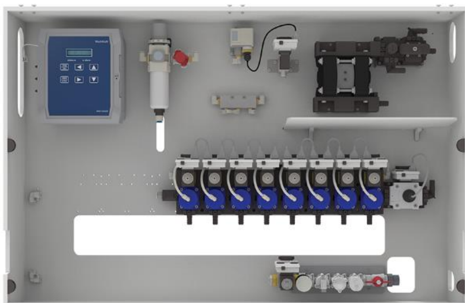
Obr. 1 – Dávkovací systém SEKO – WashMulti Air.
