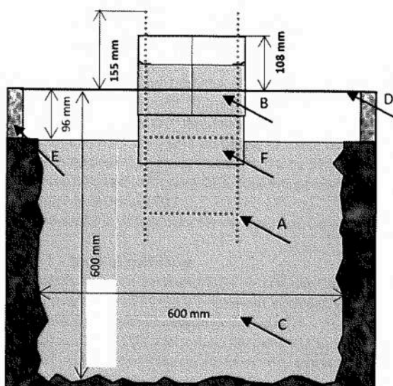
Varianta č. 3 (ovládací prvky ve výšce 1300 mm)
