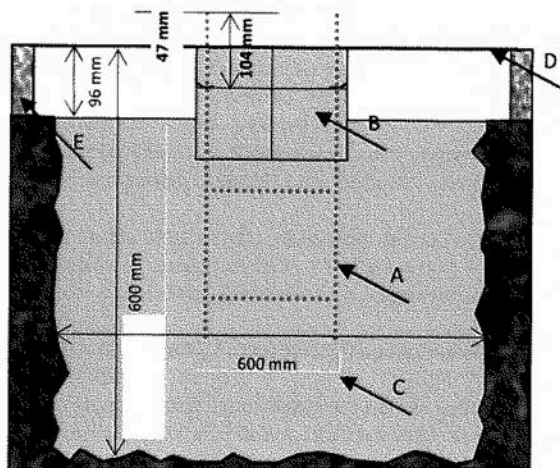
Varianta č. 1 (ovládací prvky ve výšce 1200 mm (EN15291, DDA, ADA))
