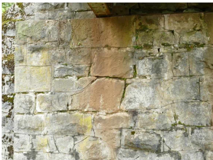
Opěra O 02: Vypadané spárování dříku
