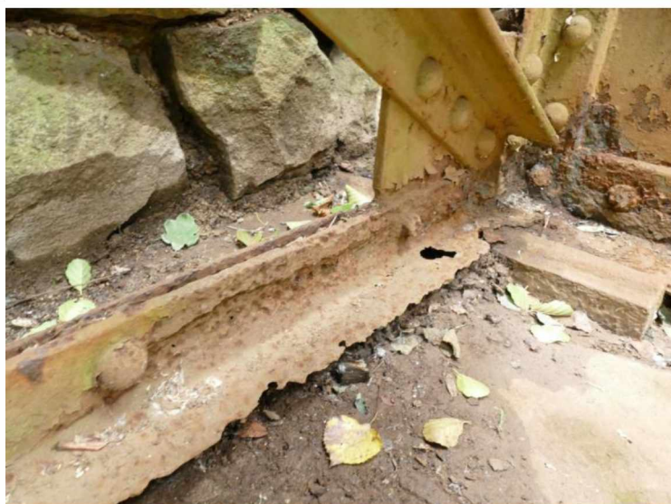
Konstrukce K 01: Korozní oslabení dolního krčního úhelníku 8. příčného ztužení
