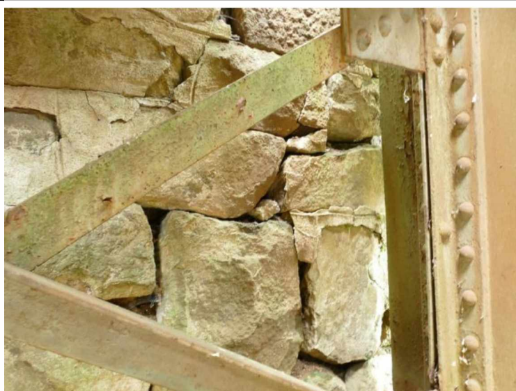
Opěra O 02: Vypadané spárování závěrné zdi
