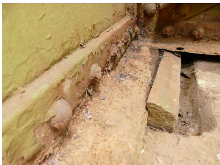
Konstrukce K 01: Zešikmené pravé ložisko na opěře O 01
