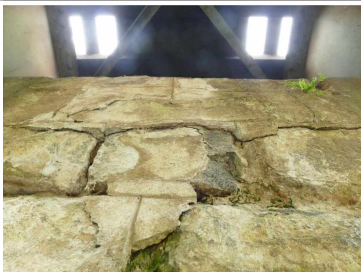
Opěra O 01: Počínající vysouvání zdiva dříku v horní části
