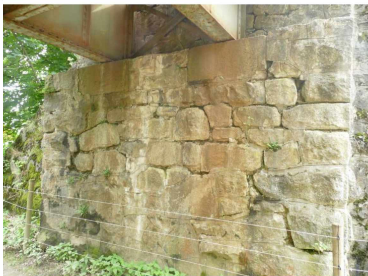
Opěra O 01: Vypadané spárování dříku
