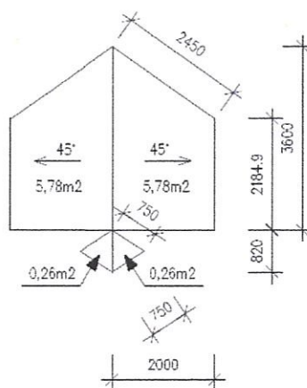
ROZVINUTÝ PŮDORYS STŘECHY VIKÝŘE (5,78m²+5,78m²+0,26m²+0,26m²=12,08m²)
