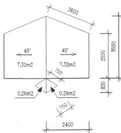
ROZVINUTÝ PŮDORYS STŘECHY VIKÝŘE (7,32m 2 +7,32m 2 +0,26m 2 +0,26m 2 =15,16m 2 )
