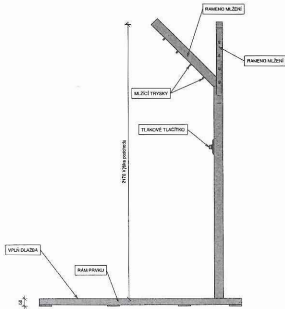
2 POHLED BOČNÍ 1 : 10
