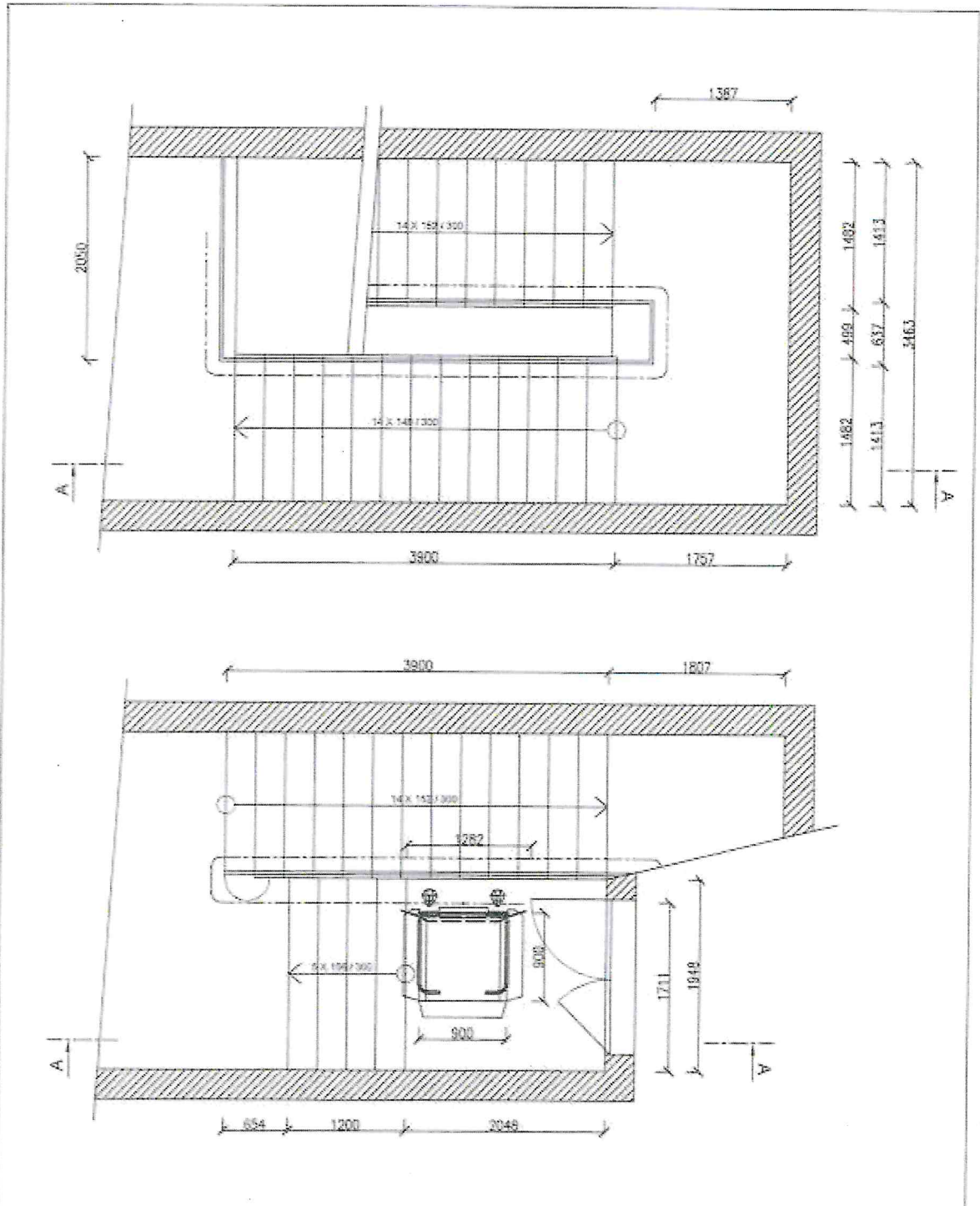
Obrázek 2: Výkres Plošina
