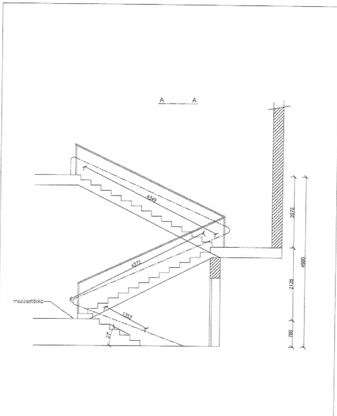
Obrázek 3: Výkres plošina
