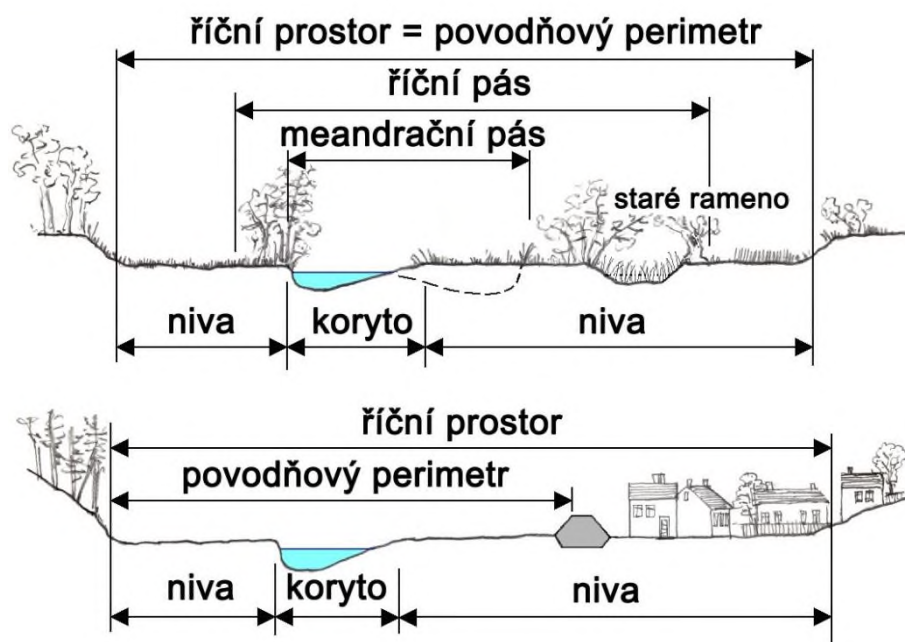
Obr. 69: Členění říčního prostoru meandrujícího vodního toku v ploché nivě. Nahoře přirozené podmínky povodňových rozlivů. Dole jsou rozlivy omezeny ochranným ohrázděním zastavěné části nivy. Převzato z Just a kol. (2020).
