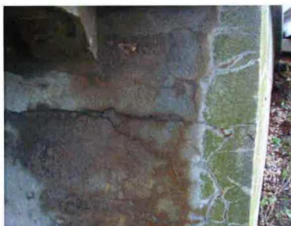
podélné trhliny a hloubková degradace betonu na čele opěry na zač.mostu
