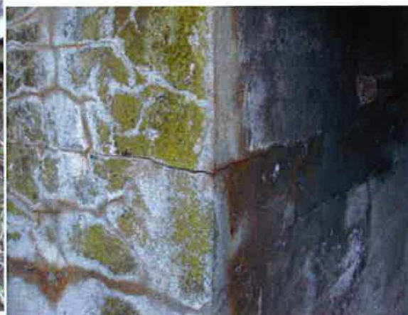
detail trhliny na čele a boku opěry na konci mostu vlevo
