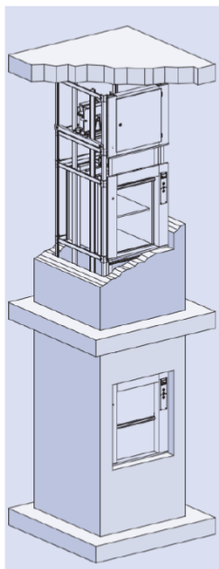
2-dílné svise posuvné dveře s parapetem
