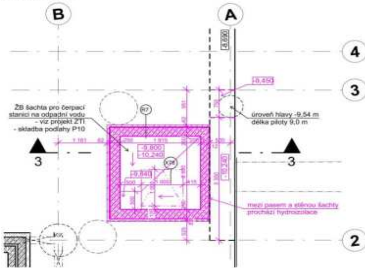
Púdorys 3.PP
