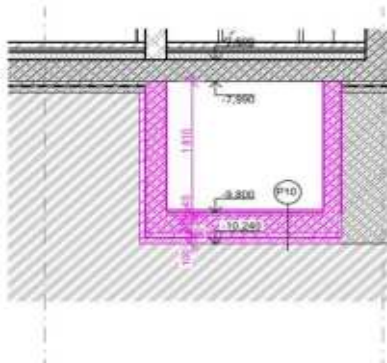
Řez 3-3'
