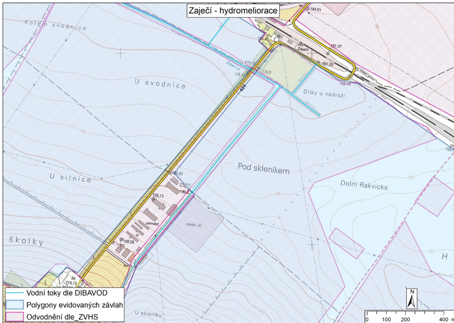
Obr. 1. Poloha evidovaných hydromelioračních staveb v rámci katastrálního území Zaječí
