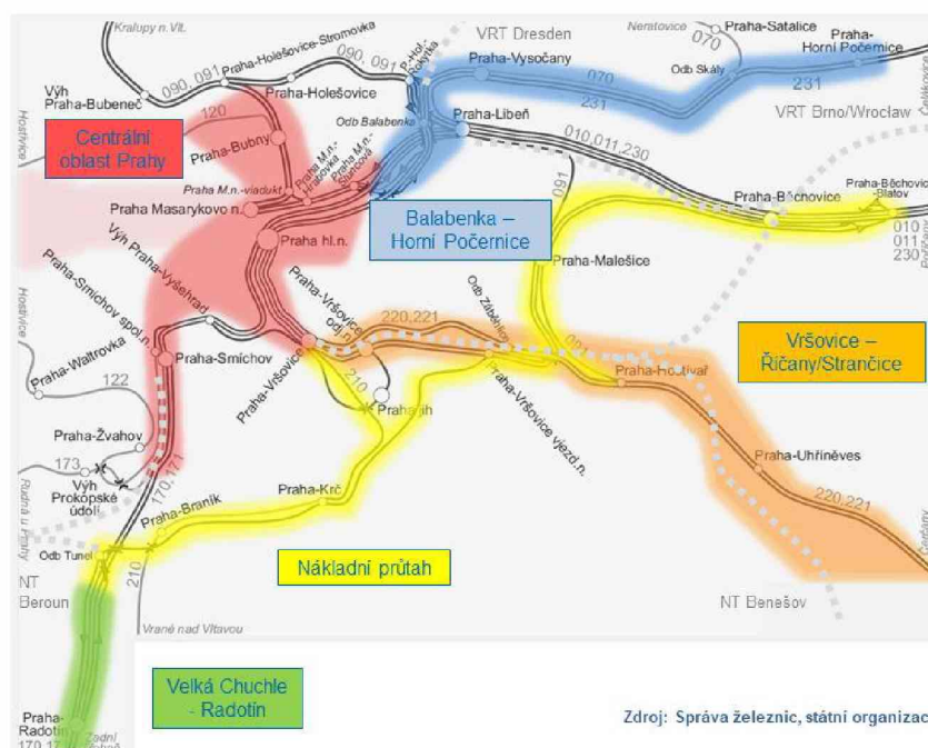
Obr. 1: Aktualizovaná přehledná situace jednotlivých oblastí železničního uzlu Praha k prověření
