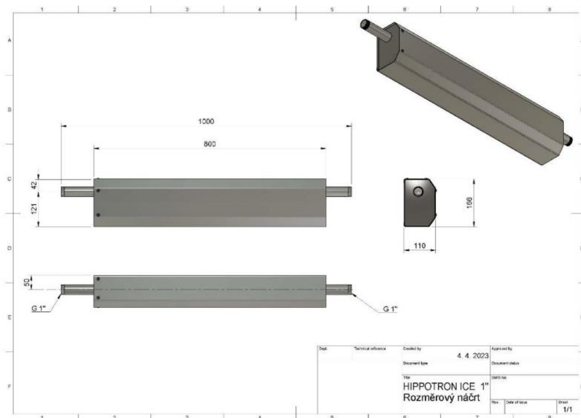
Obrázek 3 Rozměrový výkres
