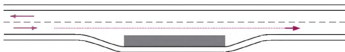
Obrázek 11 Autobusová (trolejbusová) zastávka mimo jízdniému pruh (bez fyzického oddělení - zálivová zastávka) - Typ II
