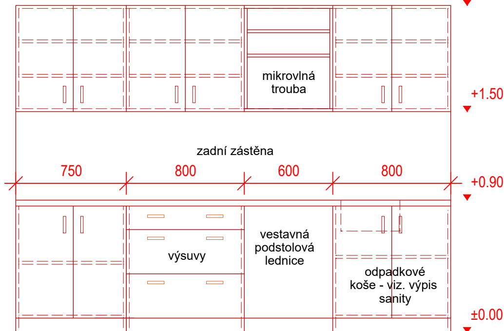
POHLED A
