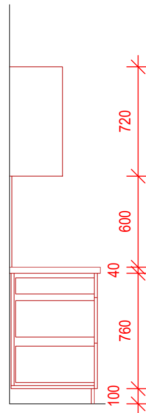
ŘEZ B-B
