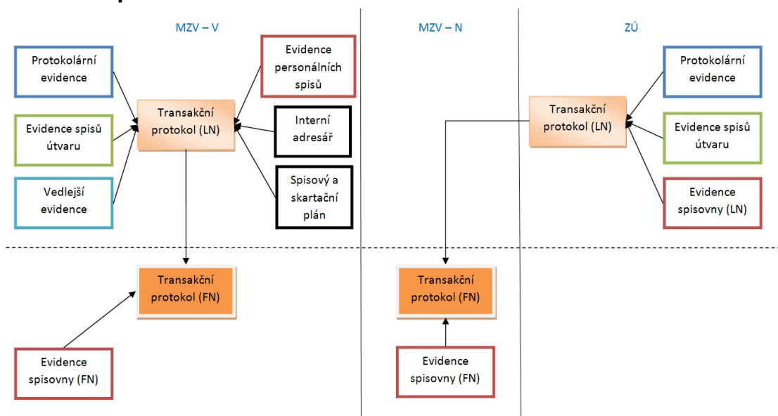
Diagram toku dat pro transakční logy
