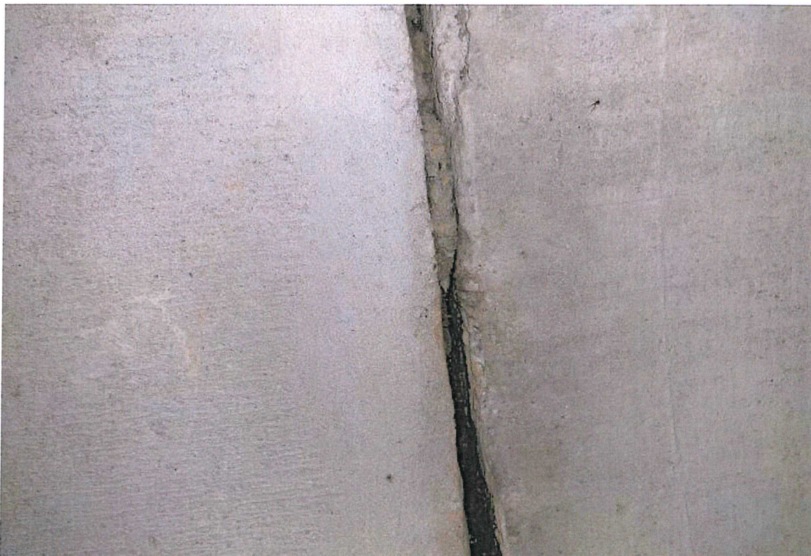
SO 02 - Sdružený objekt – detail poškození napojení potrubí DN 1200
