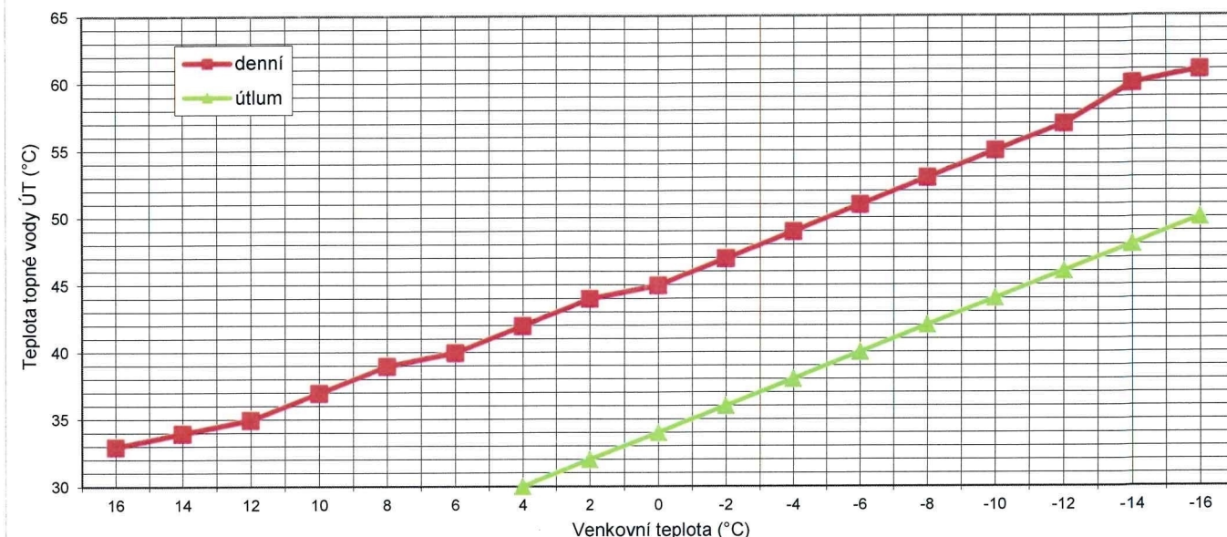
Teplotní křivka
