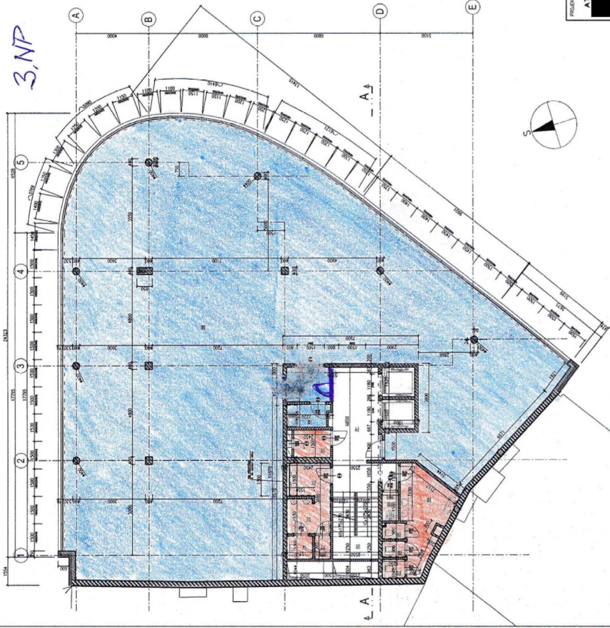
LEGENDA MÍSTNOSTI 3.NP
